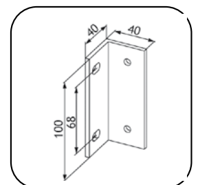
Laibungswinkel
