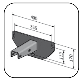
Wandkonsole (optional)
