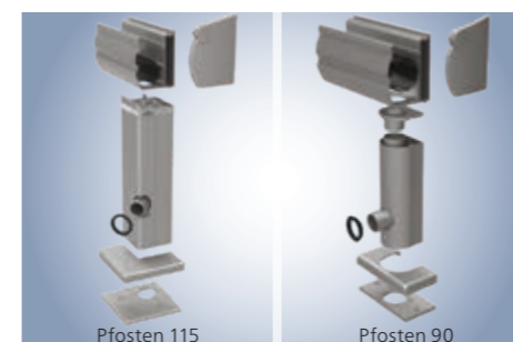
Pfosten 115
